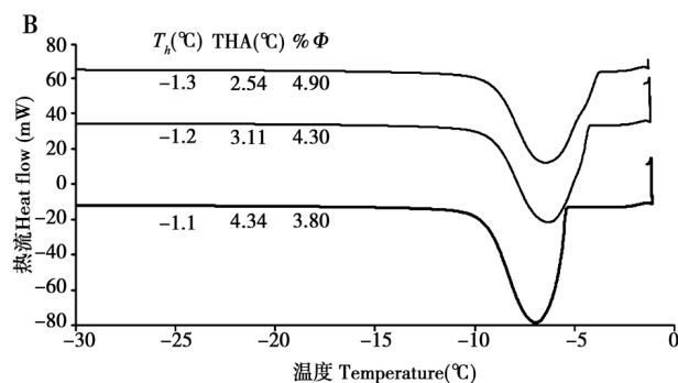
图2 黄粉虫幼虫总蛋白(A)和血淋巴(B)的热流曲线
